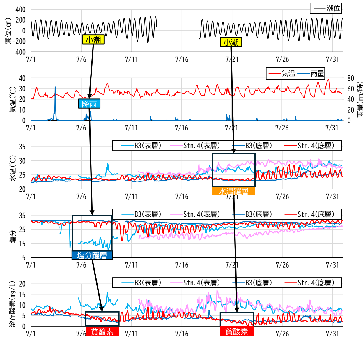
図3 貧酸素水塊形成時の潮位・気象・水温・塩分の変化（平成26年7月）
