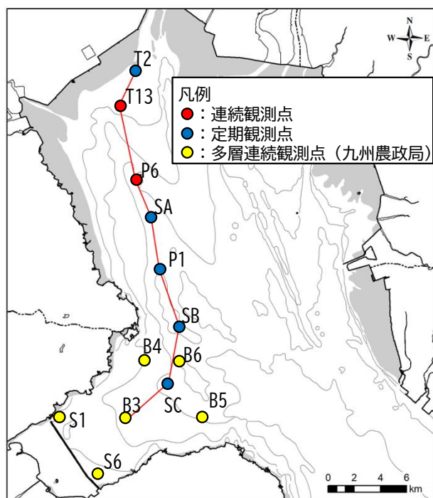
図1 有明海湾奥西側海域～諫早湾における調査位置 （観測線での調査位置）
