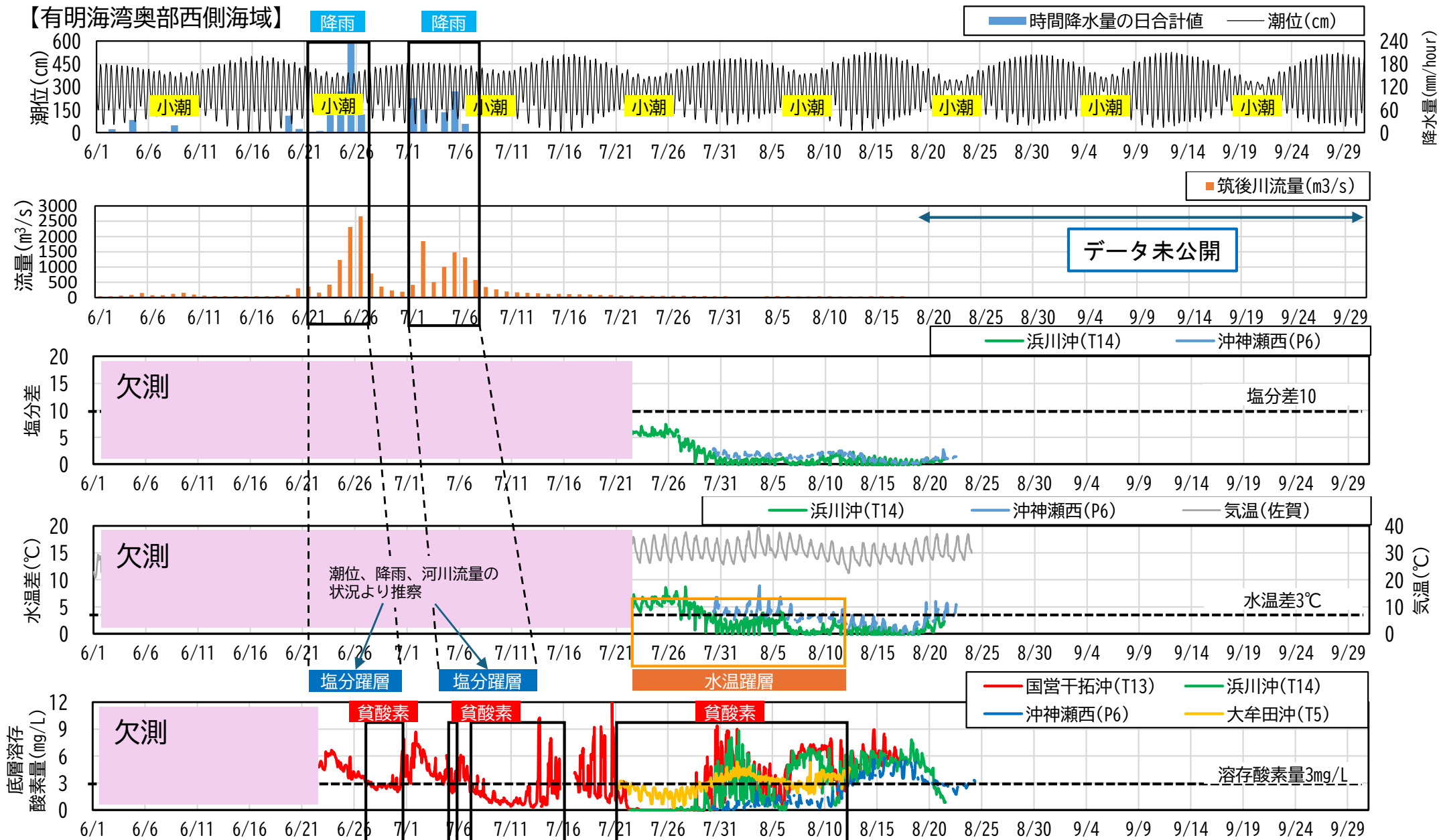
図8 有明海湾奥部西側海域における潮位、気象、塩分、水温、溶存酸素量の時系列変化（令和8年度）
