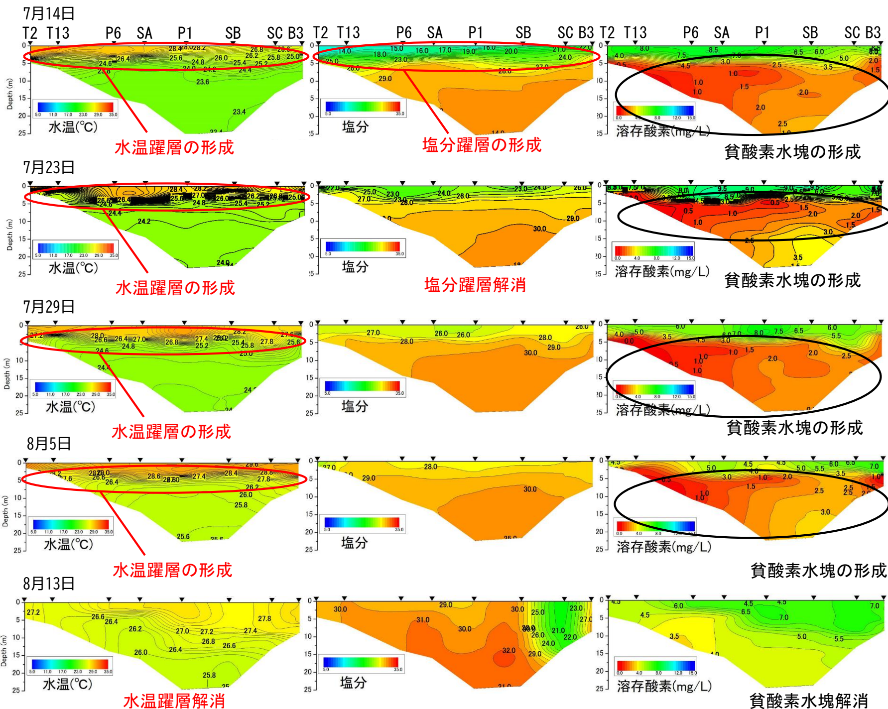
図9 貧酸素水塊の形成状況 (令和8年) 出典：水産技術研究所 環境・基盤部門 沿岸生産システム部
