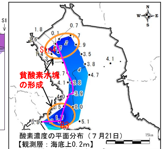
図6 海底上0.2mの溶存酸素量平面分布（平成26年7月21日）
