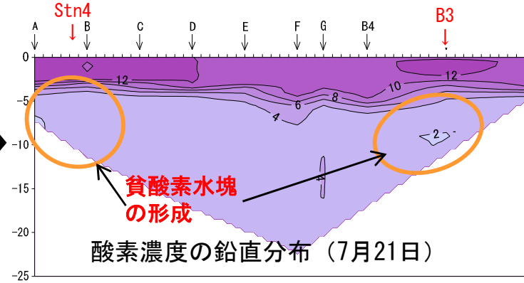
図5 貧酸素水塊の形成状況（平成26年7月14日→7月21日）
