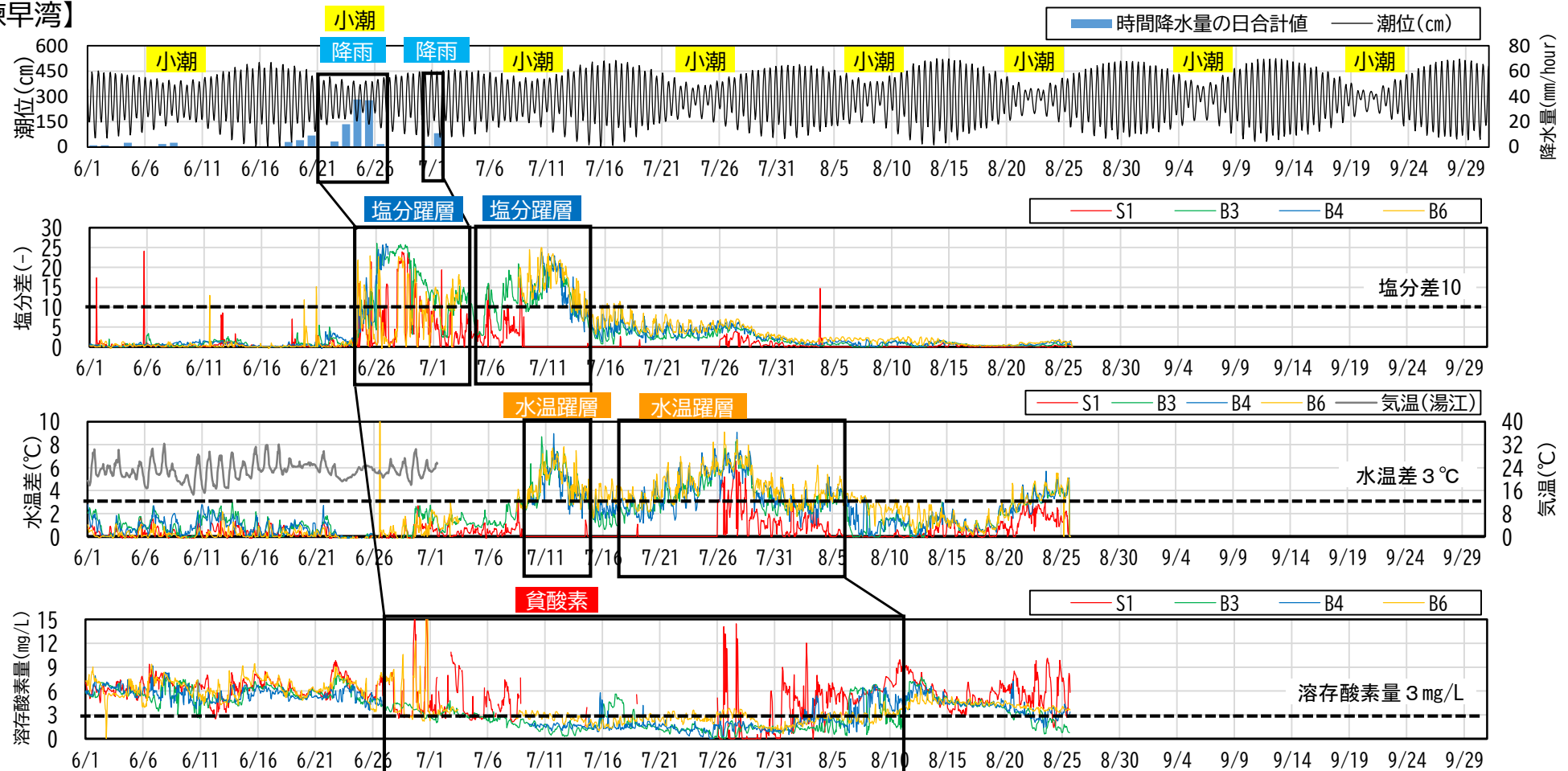
図7 諫早湾における潮位、気象、表層と底層の塩分差・水温差、溶存酸素量の時系列変化（令和8年度）
