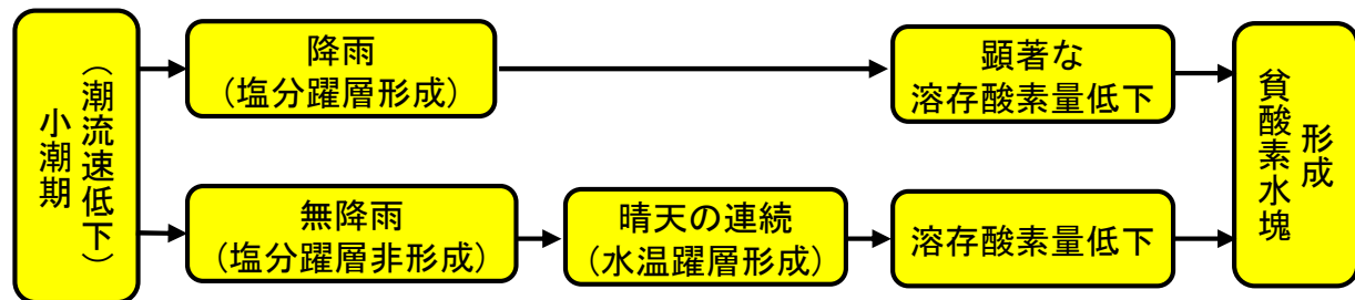
図2 貧酸素水塊形成のメカニズム
