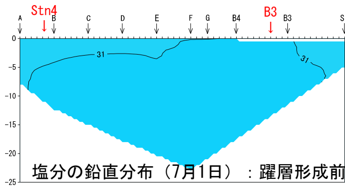
図4 水温躍層と塩分躍層の形成状況（平成26年7月1日、7月14日、7月21日）
