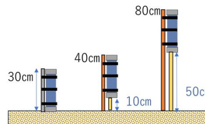
ネトロンパイプを用いた設置高さの検討
