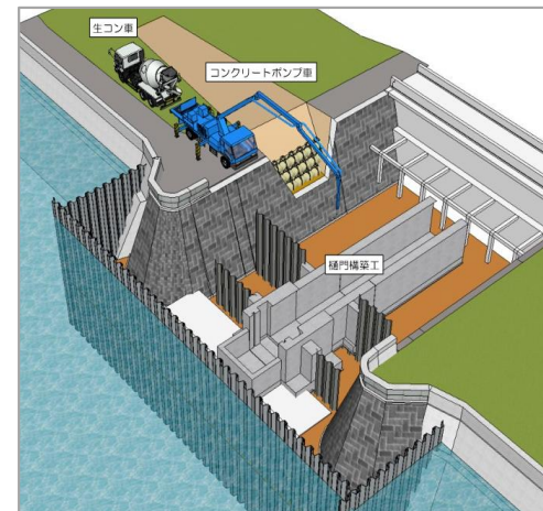
樋門工事概要図
