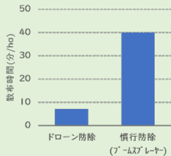
（水稻）ドローンの活用により除草剤散布時間は、慣行の18%に短縮。粒剤散布など汎用性が期待できる(5～7月)
