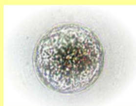
受精卵
