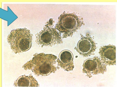
卵子
