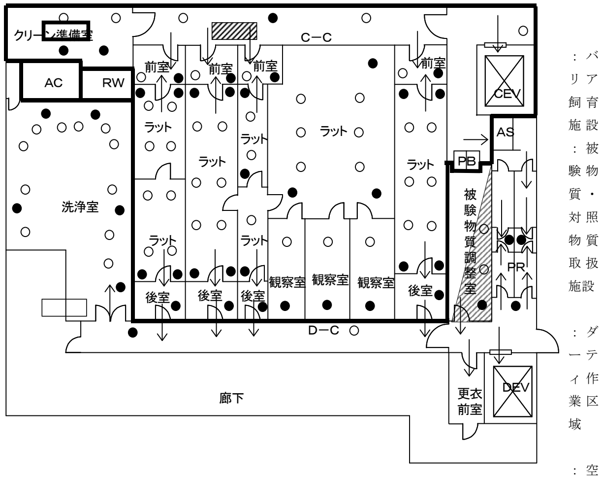
(例) 施設の空調概略図
