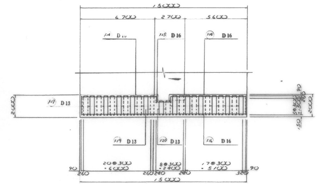
2-2断面図 S=1:100
