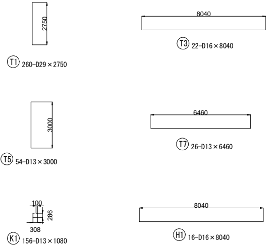
底版 1面 (20m2×2) 当たり
