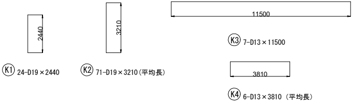
隔壁 W=1200 1面当たり
