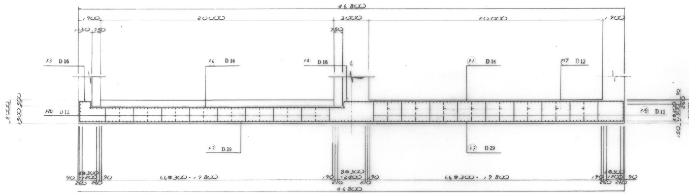
1-1断面図 S=1:100
