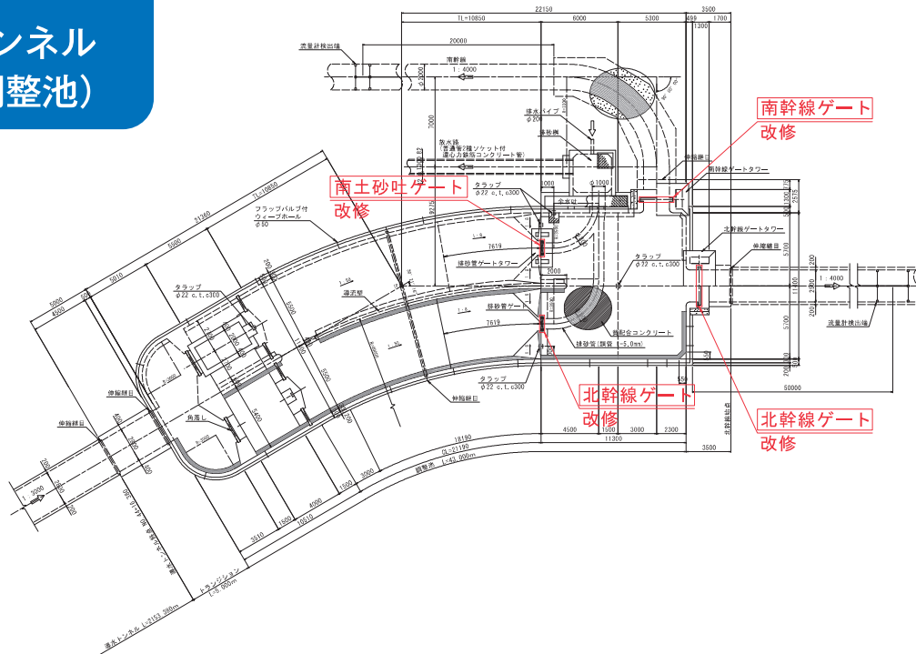
主要構造図 導水トンネル（南北調整池）
