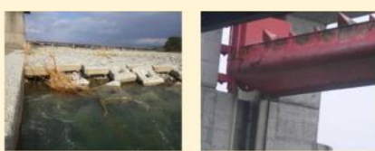
【護床ブロック】 流失、不同沈下 【ゲート設備】 表面劣化
