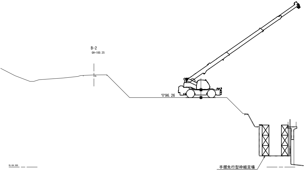
横断面図 S=1:200
