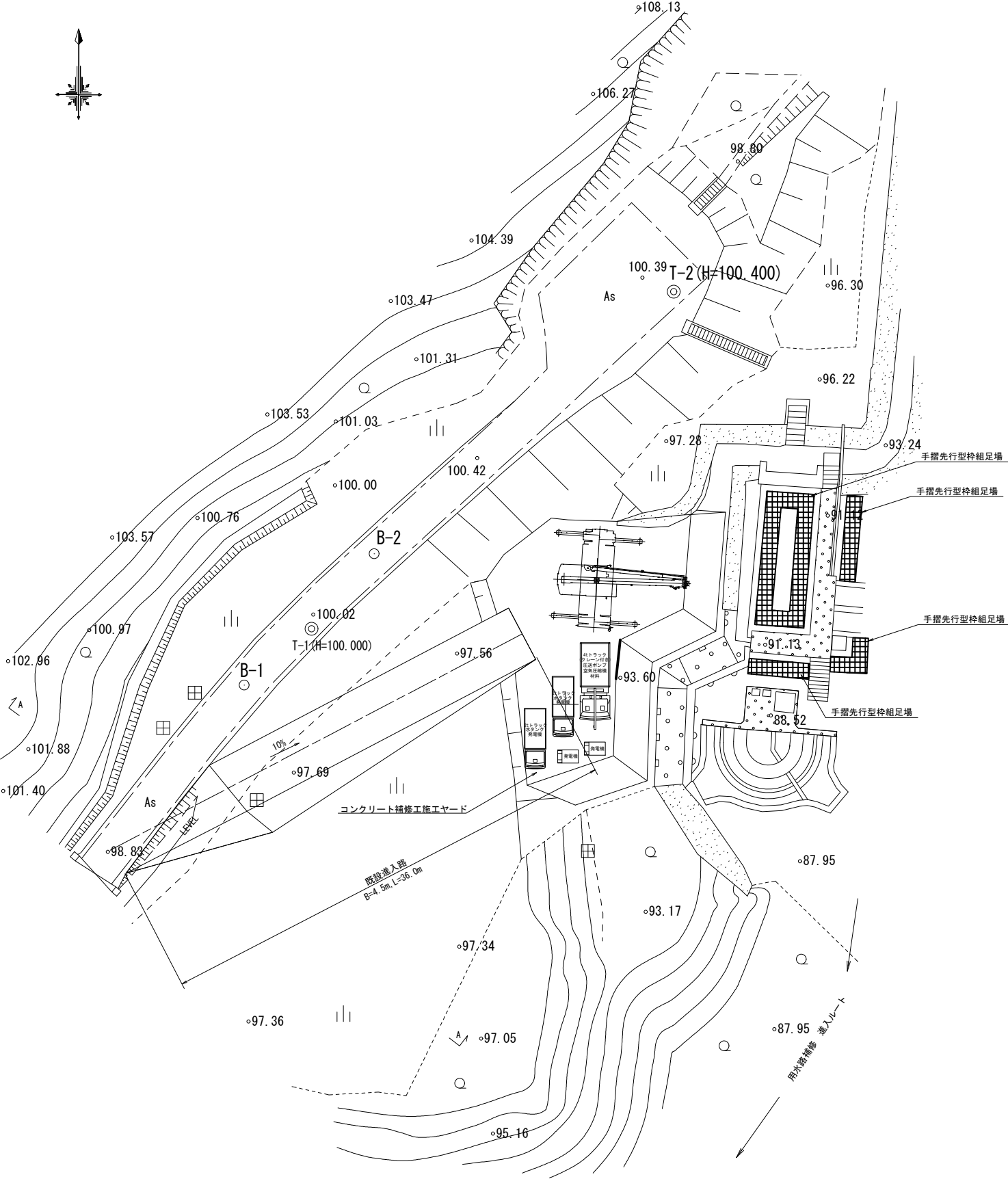
平面図 S=1:200
