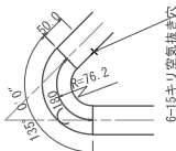
"B"詳細図
