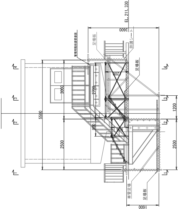
正面図
