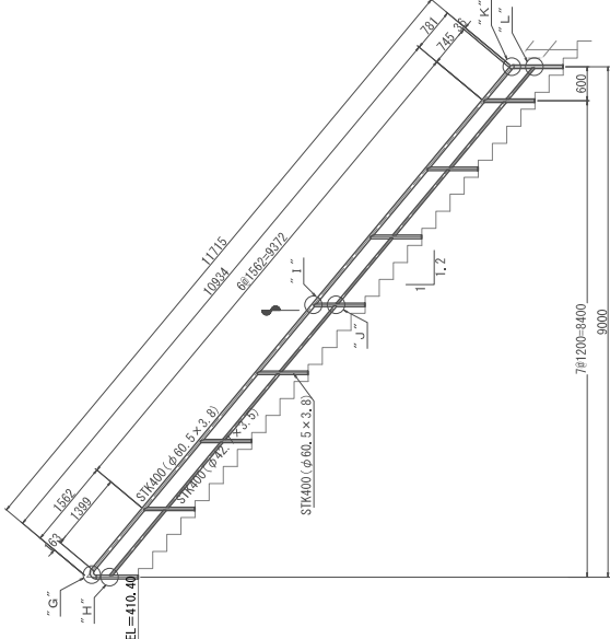
B区間手摺詳細図
