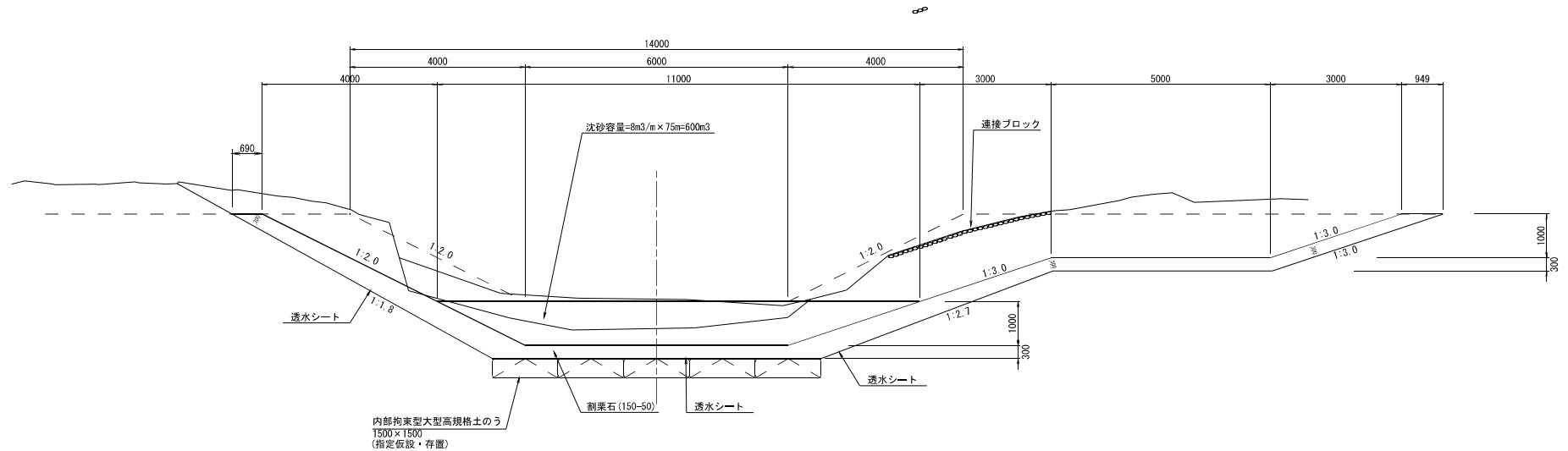
断面図
