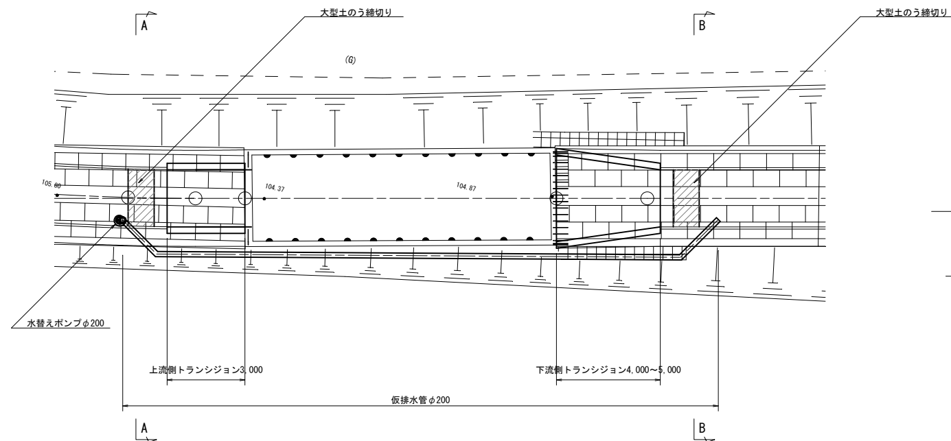
平面図 S=1:100
