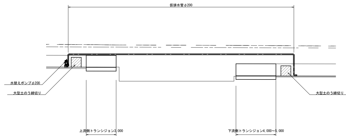
縦断図 S=1:100
