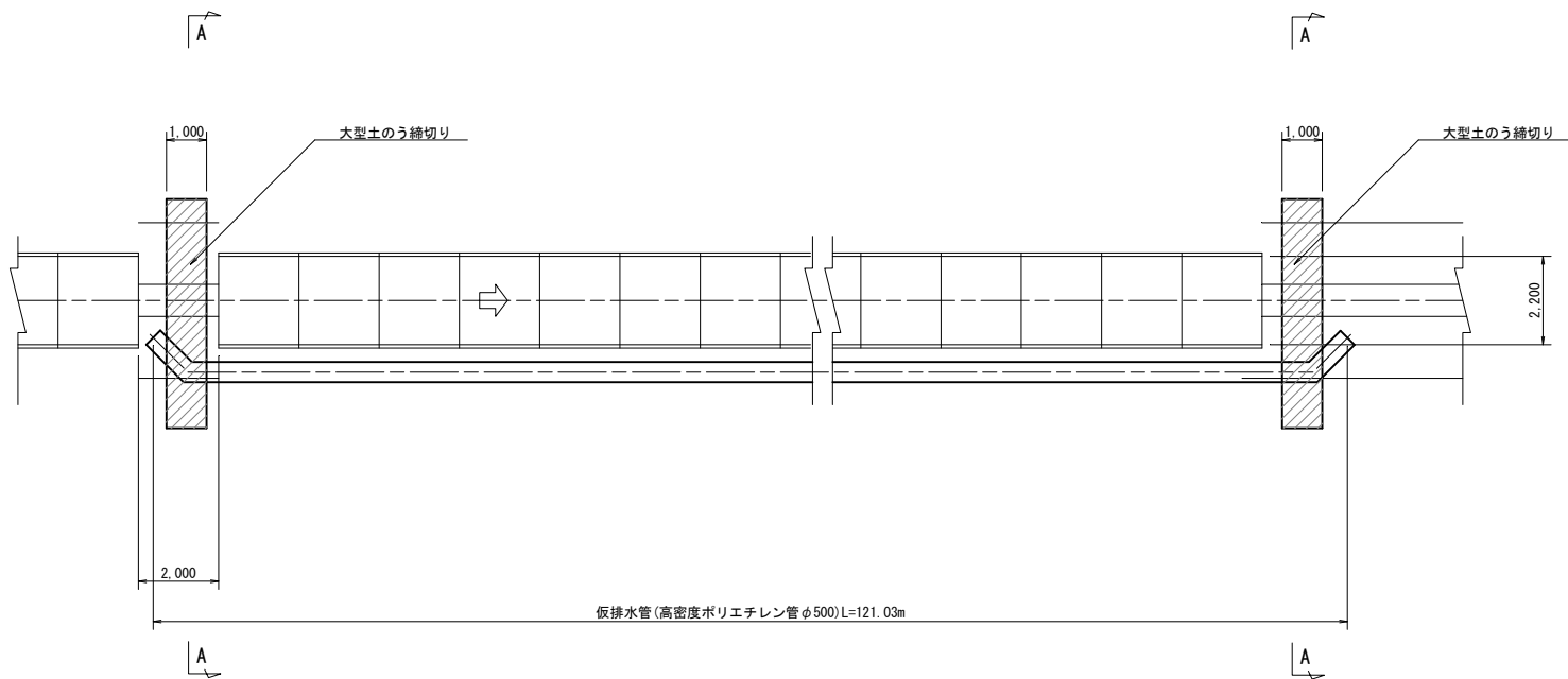
平面図 S=1:100
