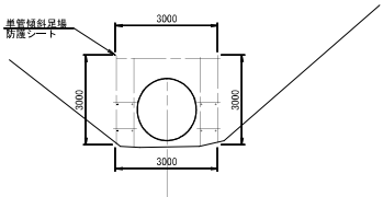
標準断面図
