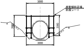
標準断面図
