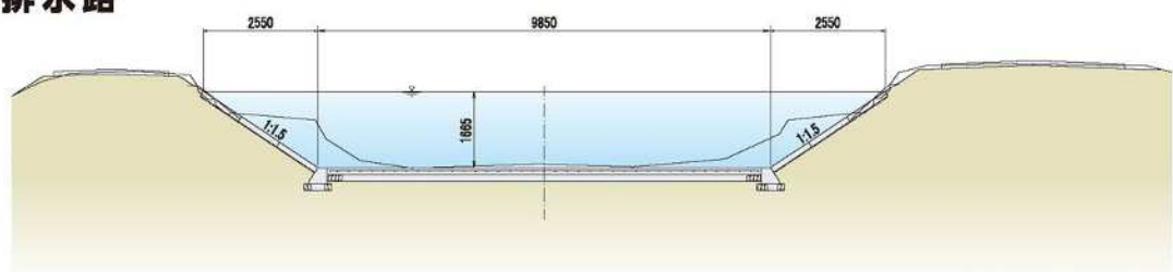
農道区間 標準断面図
