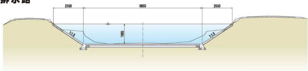
農道区間 標準断面図
