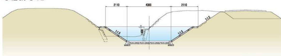
1型水路 標準断面図
