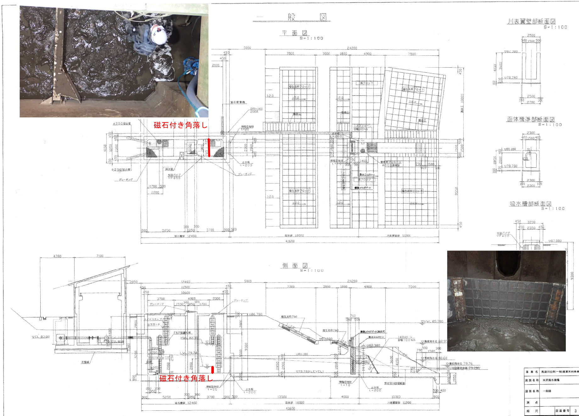
参考図 馬淵川沿岸地区 米沢揚水機場一般図
