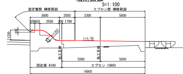
縦断面図
