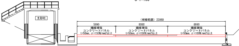
正面図 S=1:100
