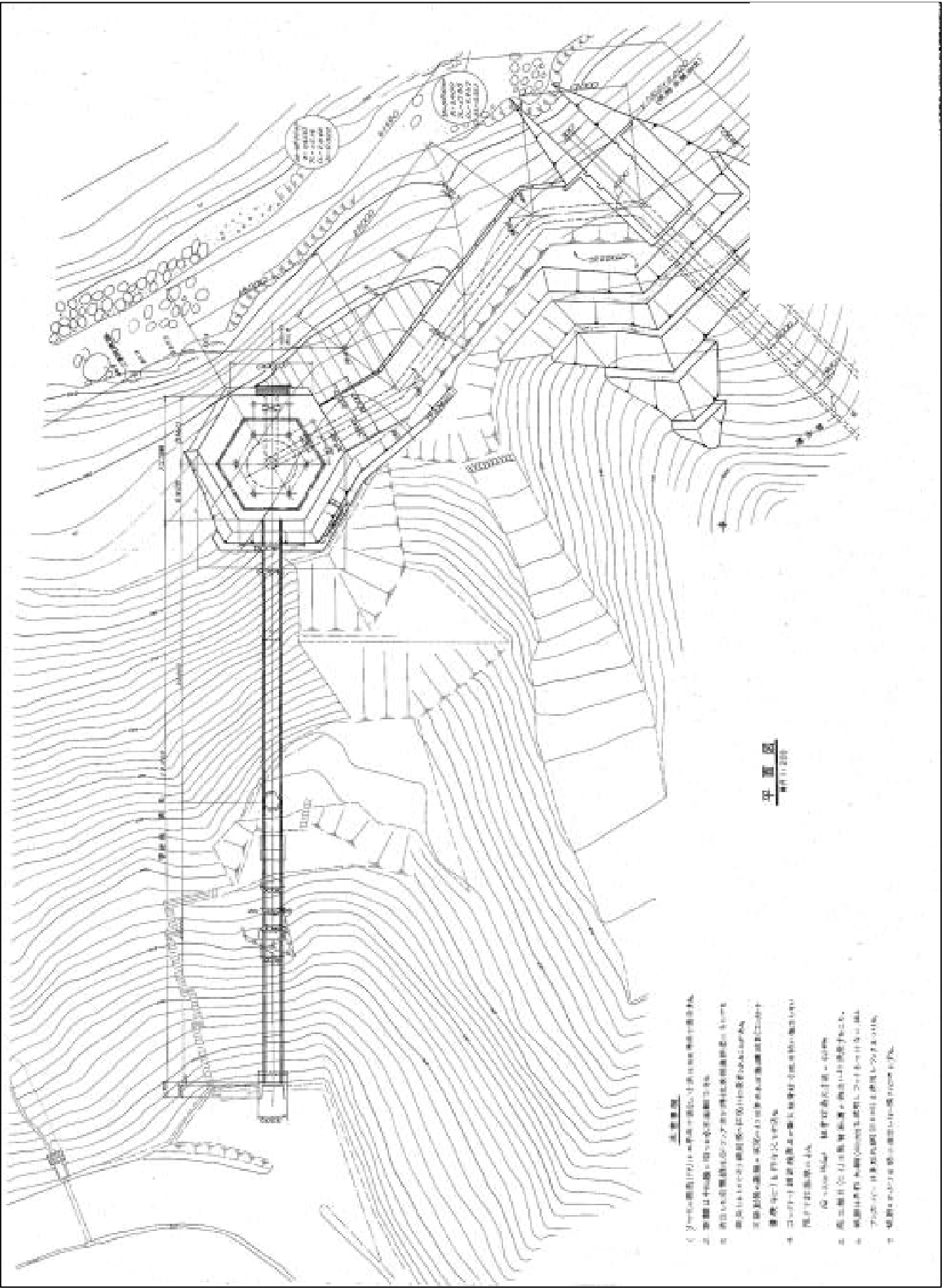
荒砥沢ダム 取水設備平面図
