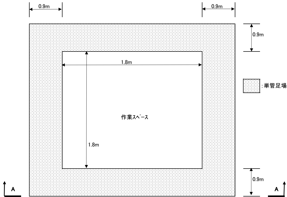
平面図
