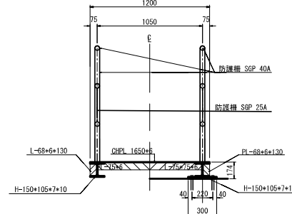
管理橋断面図
