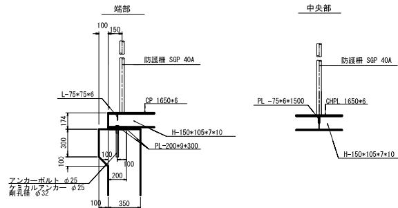
手摺取付詳細図
