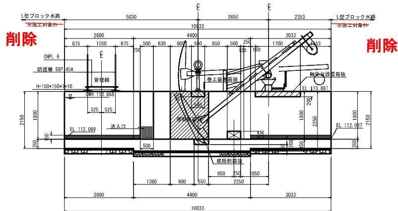
縦断面図
