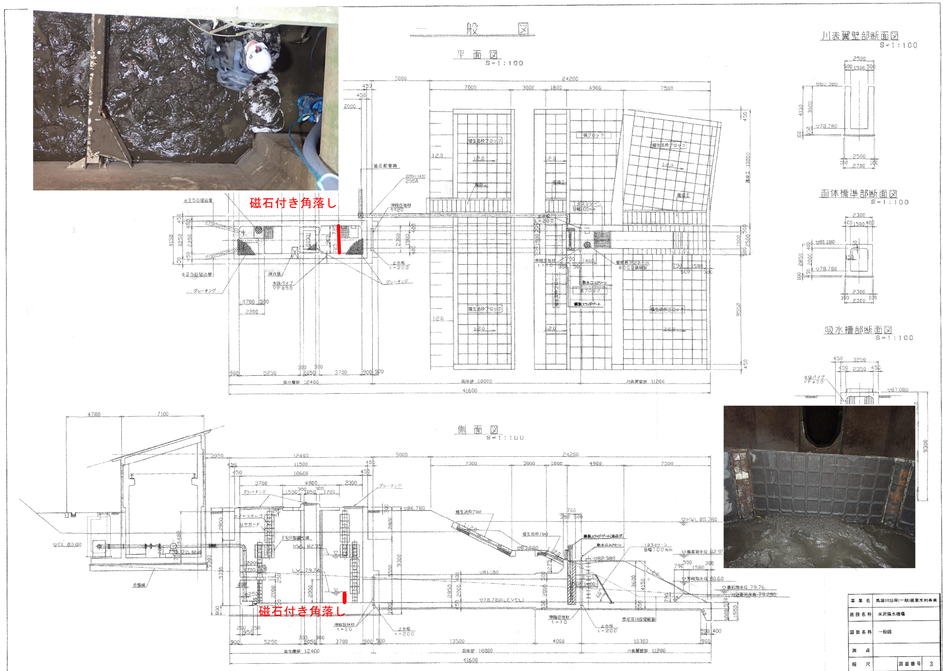
【参考図】 2 1. 馬淵川沿岸地区 米沢揚水機場一般図
