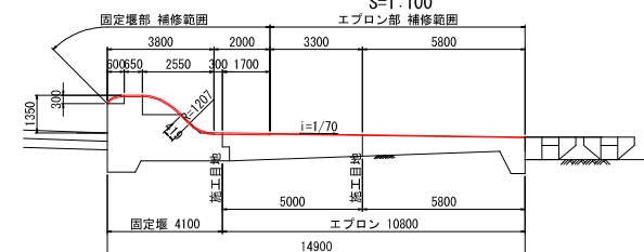
縦断面図
