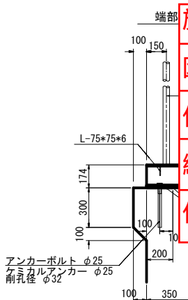
手摺取付詳細図
