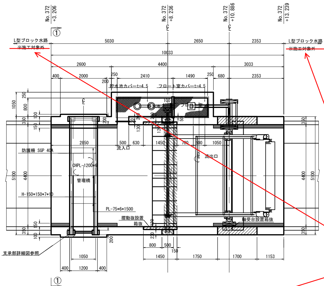
縦断図
