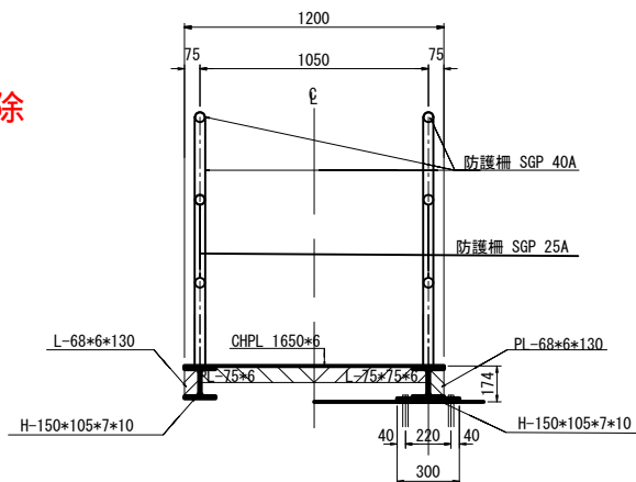
管理橋断面図
