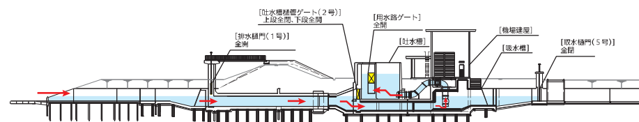
【排水時のゲート操作】
