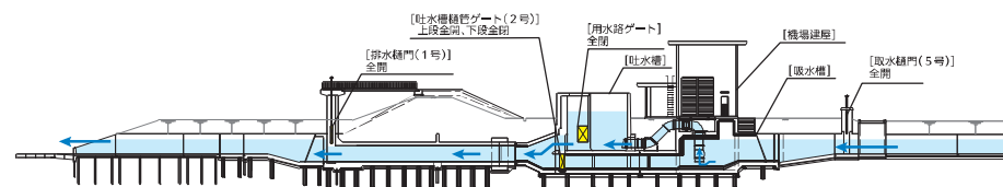
【排水時のゲート操作】
