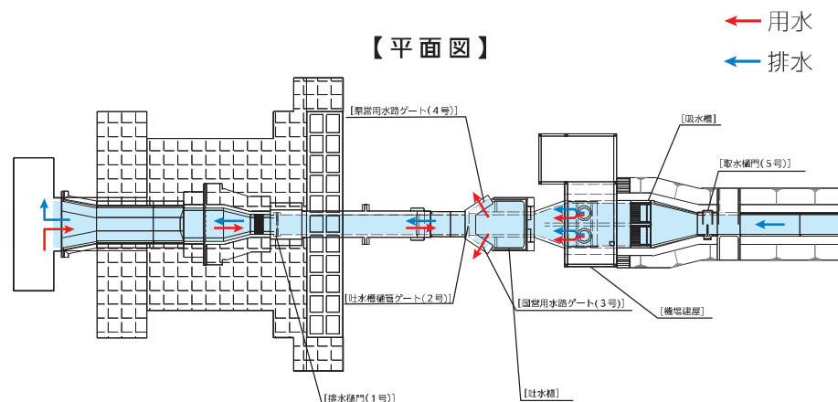
【用水時のゲート操作】
