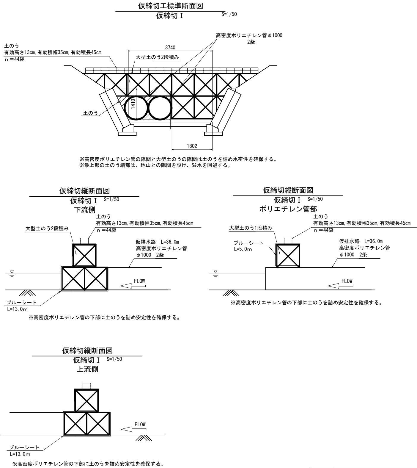
仮締切工Ⅰ（Ⅲ型水路） 2-N0, 15+18.00～2-N0, 18+18.00 L=90.00m
