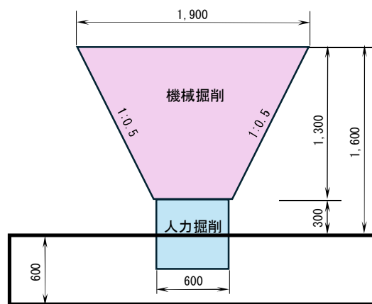
掘削断面図(縦断方向)
