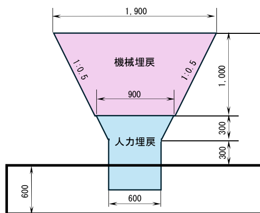
埋戻断面図(縦断方向)
