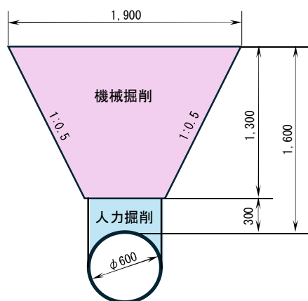
掘削断面図(横断方向)
