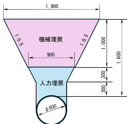
埋戻断面図(横断方向)
