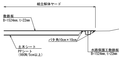
(参考図) 分解組立ヤード 断面図 S=1:100
