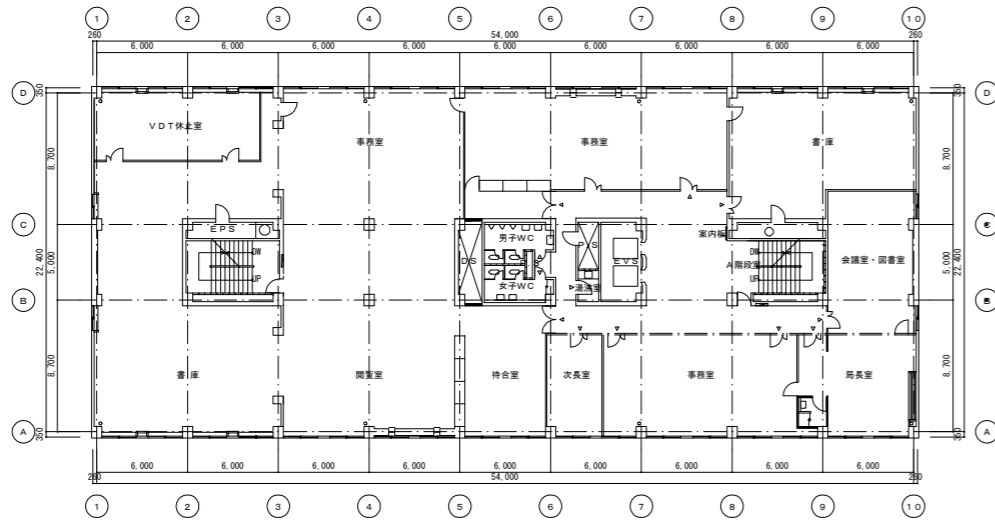
2階平面図
