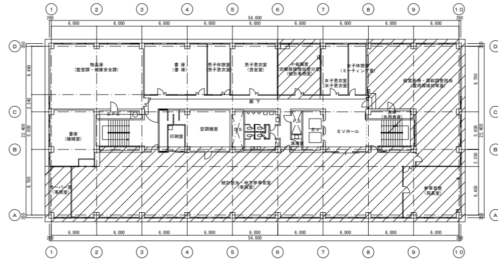
5階平面図 ※( )内は改修前室名
