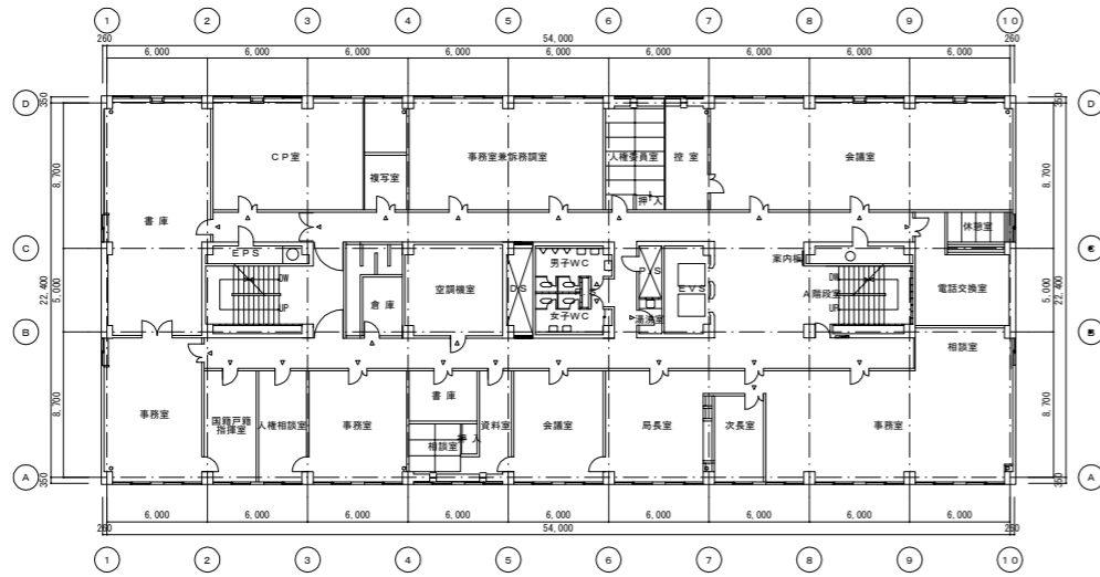
3階平面図
