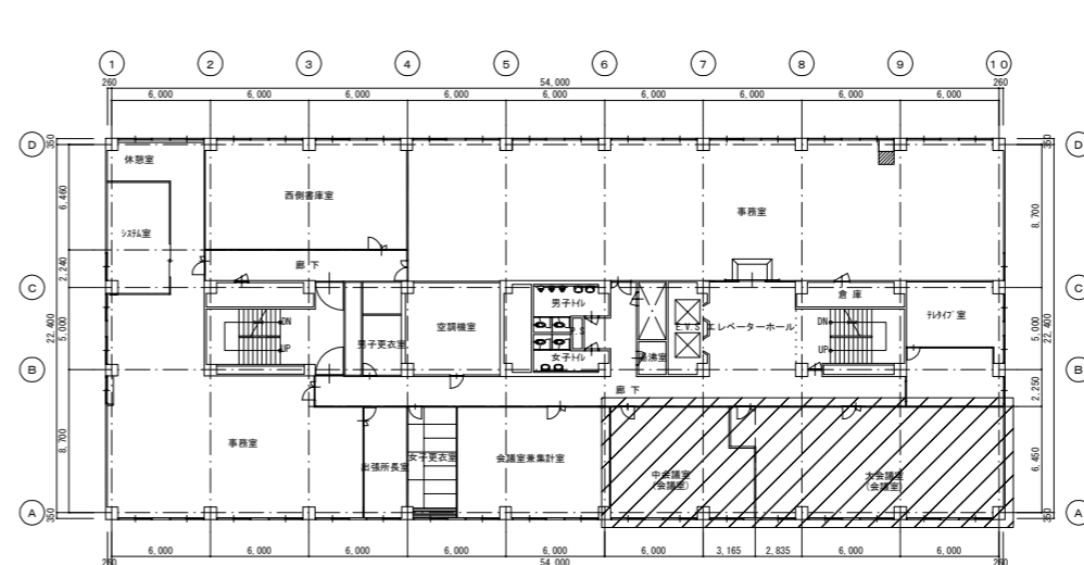
4階平面図 ※( )内は改修前室名
