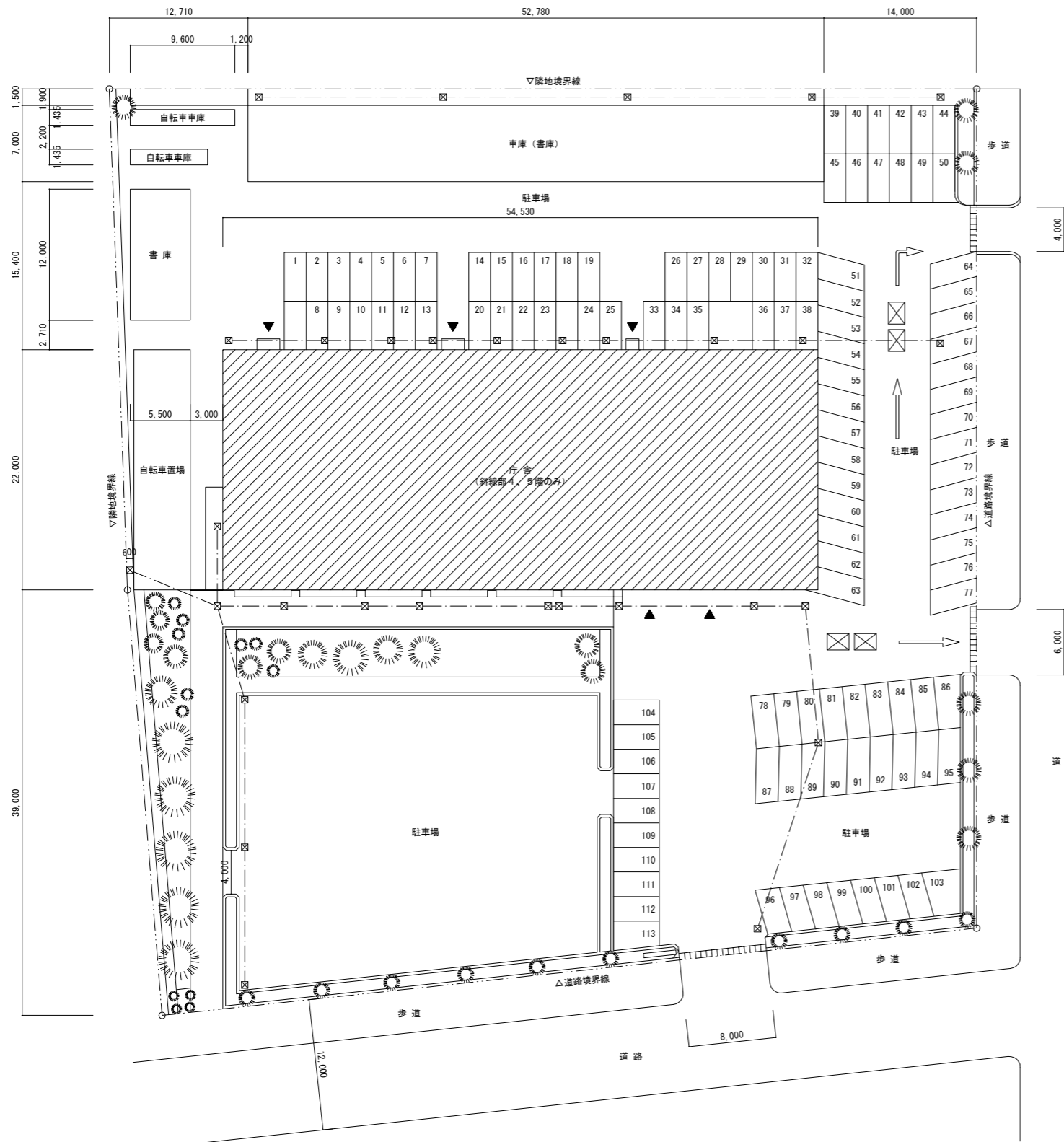
配置図 1 : 250
