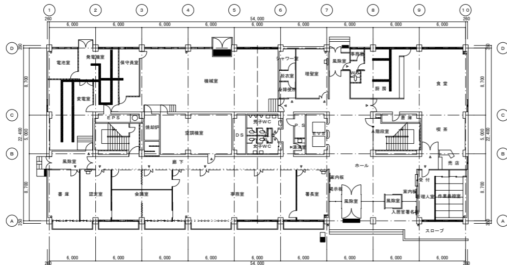
1階平面図
