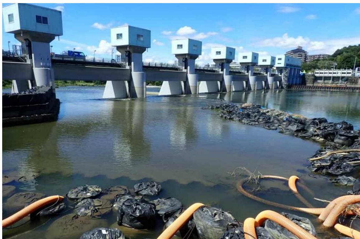
頭首工全景（左岸側から撮影）
