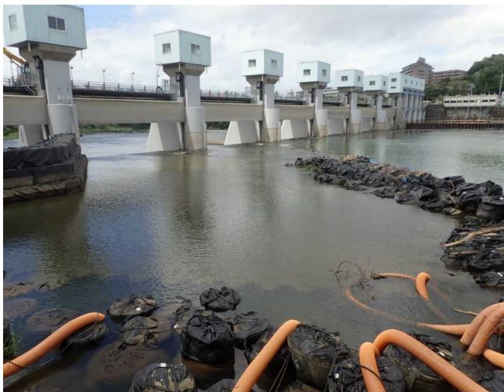
頭首工全景（左岸側から撮影）
