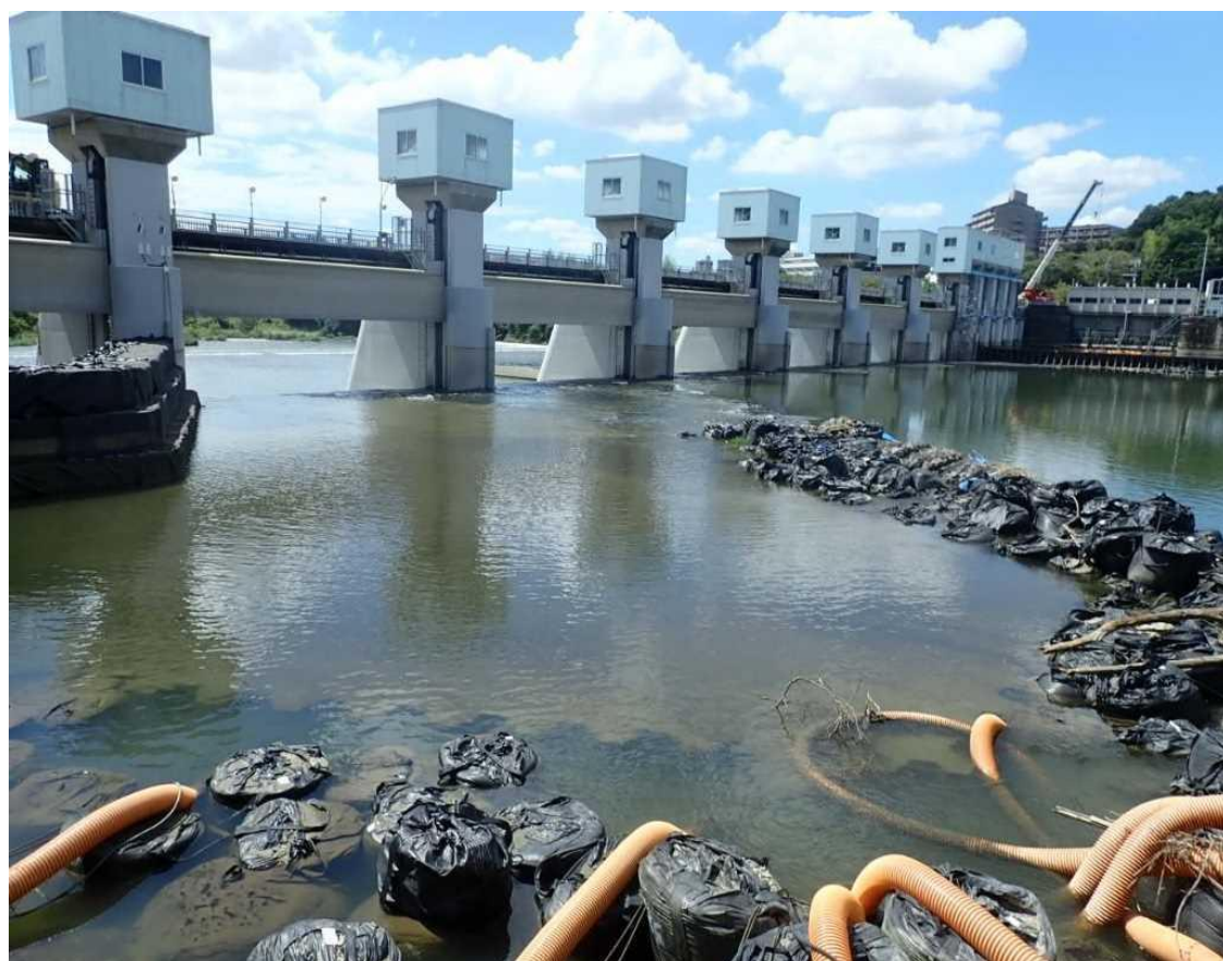
頭首工全景（左岸側から撮影）
