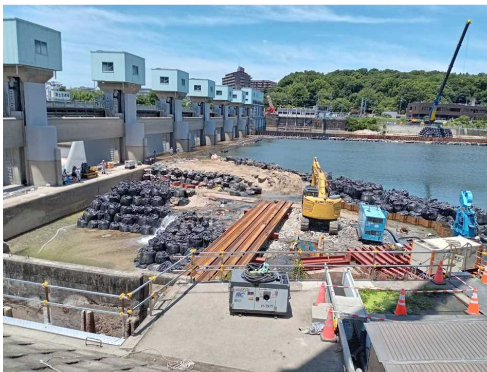
頭首工全景（左岸側から撮影）
