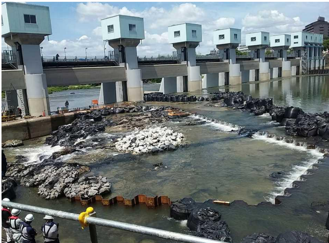
頭首工全景（左岸側から撮影）
