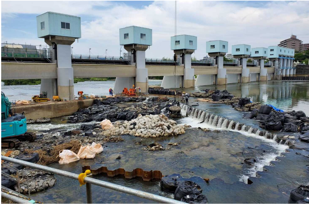
頭首工全景（左岸側から撮影）
