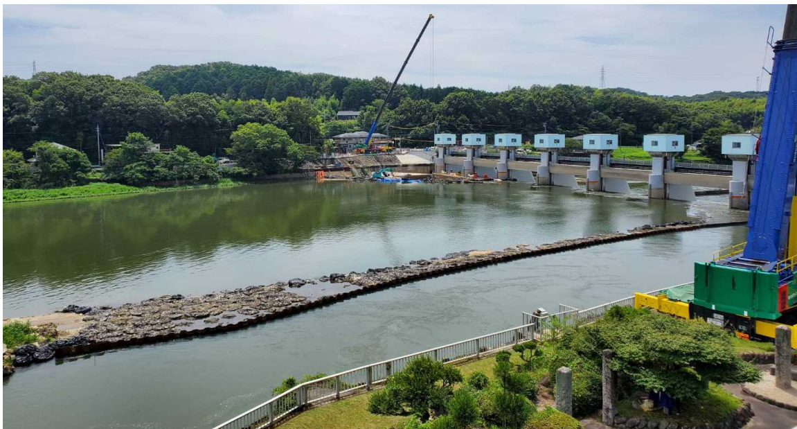
頭首工全景（右岸側から撮影）
