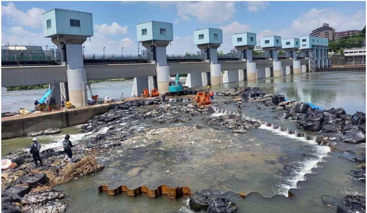
頭首工全景（左岸側から撮影）
