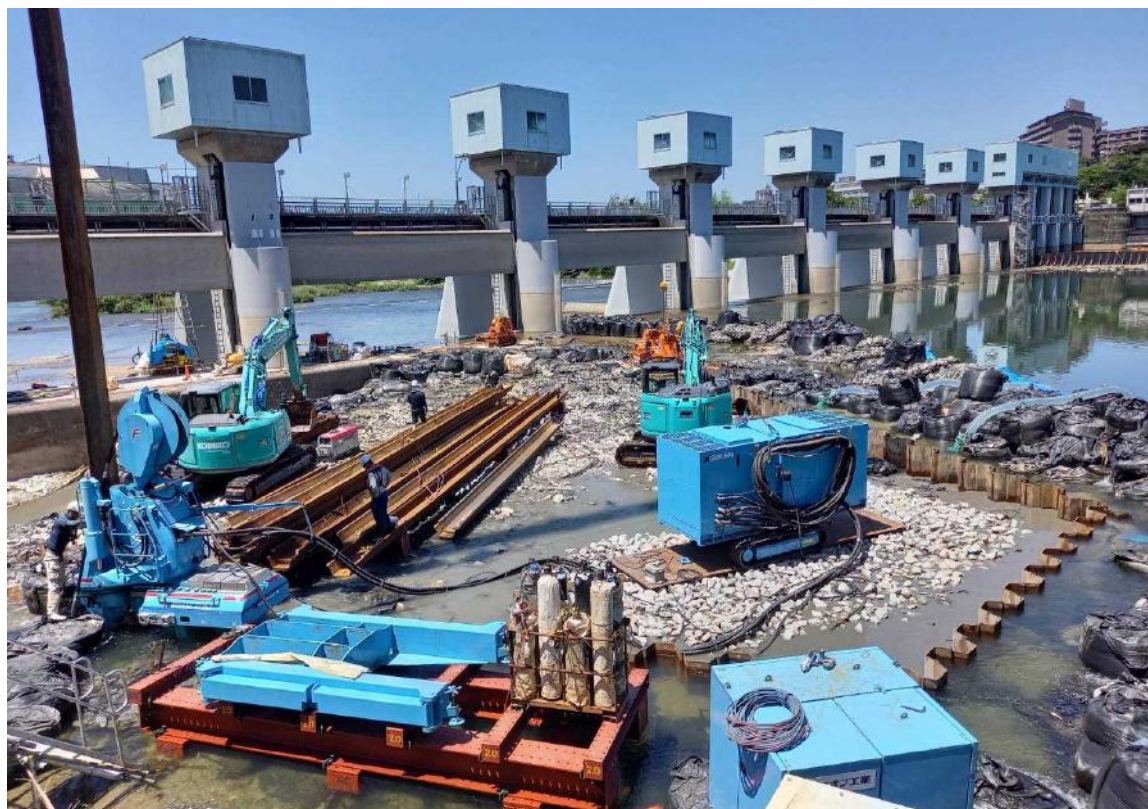
頭首工全景（左岸側から撮影）
