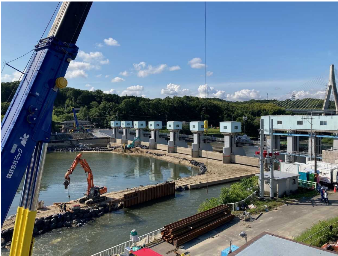
頭首工全景（管理所側から撮影）
