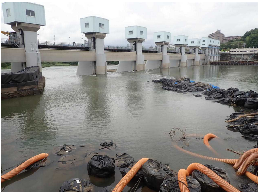
頭首工全景（左岸側から撮影）
