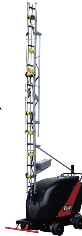
静電噴口防除ロボット
