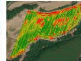
圃場内の場所ごとに計測される収量及び水分データから作成される収量マップ（次期作の施肥設計に活用）
