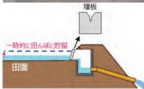
田んぼダムの取組
