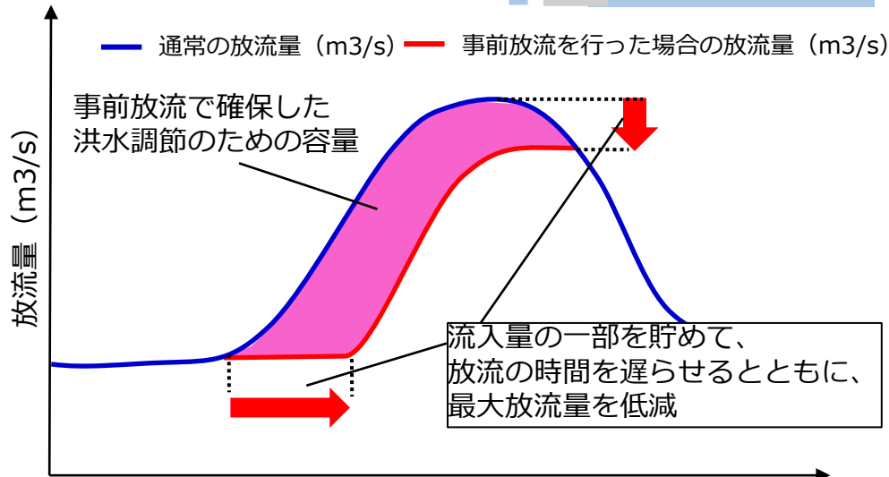
事前放流による容量確保のイメージ図 時間 (h)
