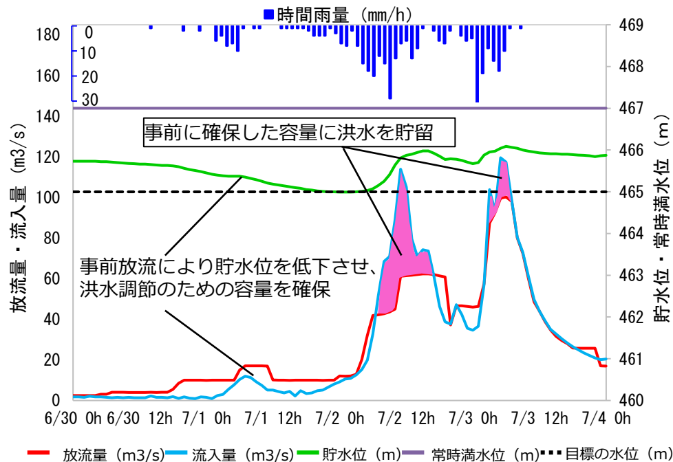
羽布ダムのハイドログラフ
