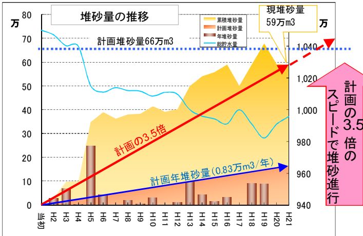
安濃ダム堆砂状況(堆砂厚7m)
