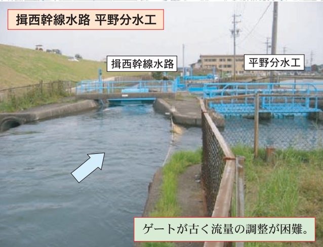
揖西幹線水路 平野分土工
